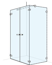
Porte battante en 2 parties version murale avec paroi latérale
