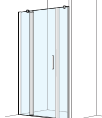
Porta girevole con elemento fisso e parete laterale allineata
