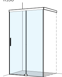
Porta scorrevole a 2 elementi con parete laterale lato elemento fisso
