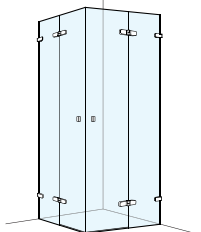
Doccia ad angolo con porte a battenti ed elementi fissi
